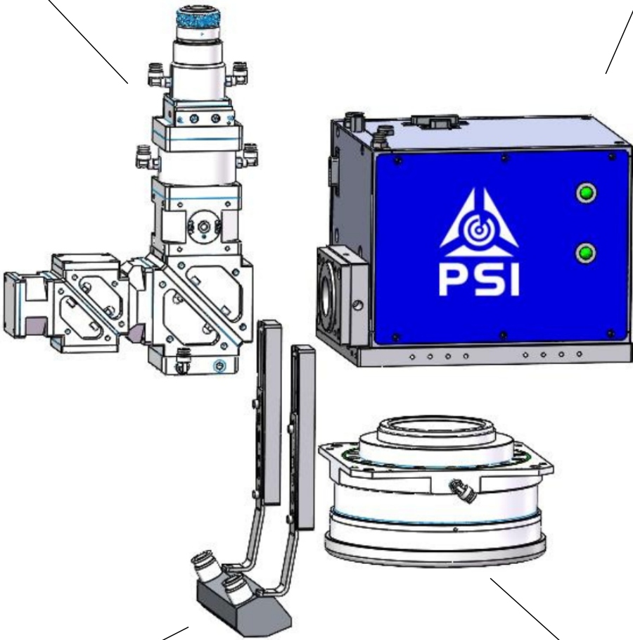
F-Theta-Objektiv
