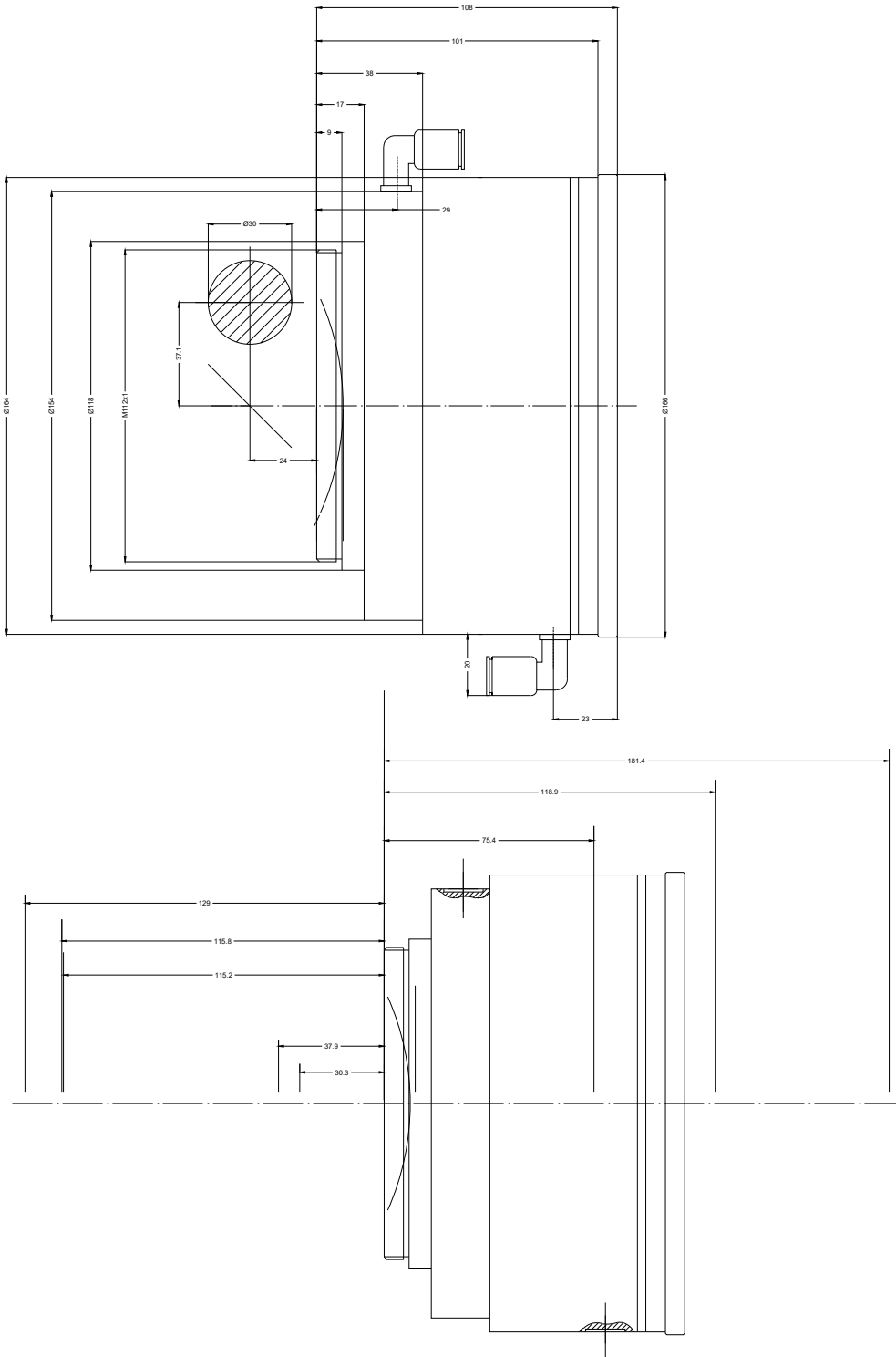
F-Theta-Objektiv
